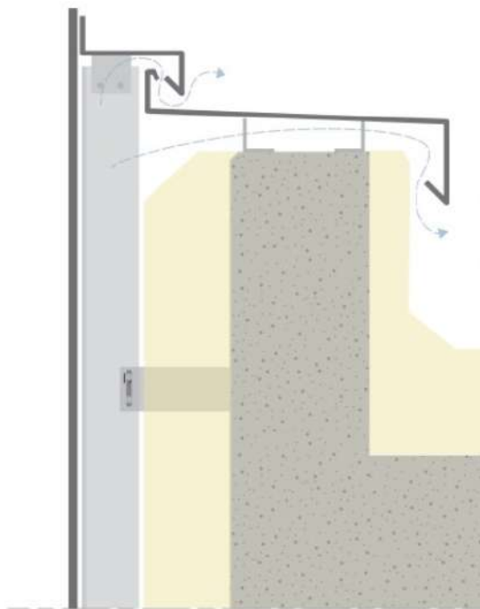
Рисунок 11: Парапет заподлицо
